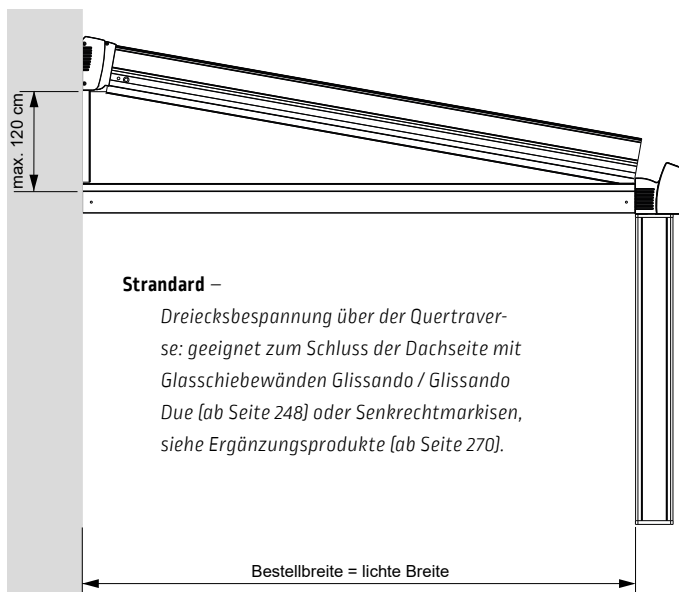
Grundprofil
