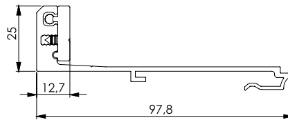
Grundprofil M2020
